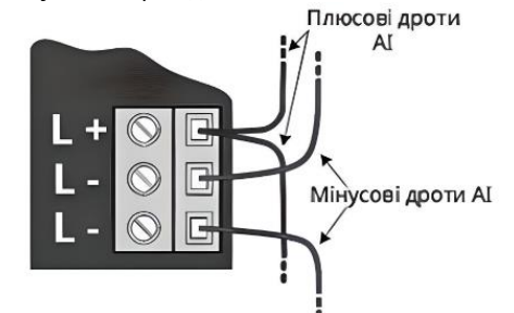
Рисунок 2 - Підключення провідників АІ СПСА до клем АІ панелі
