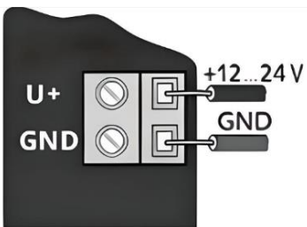
Рисунок 3 - Підключення входу живлення
