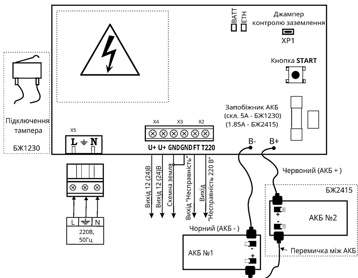
Рисунок А.2 – Підключення входів та виходів
