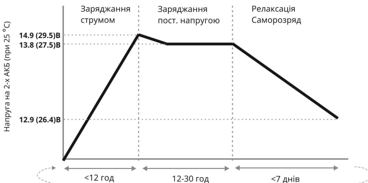
Рисунок 2 – Цикли роботи зарядного пристрою
