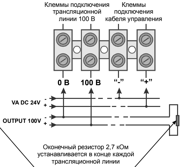
Схема подключения громкоговорителя с вмонтированным регулятором громкости к трансляционной линии
