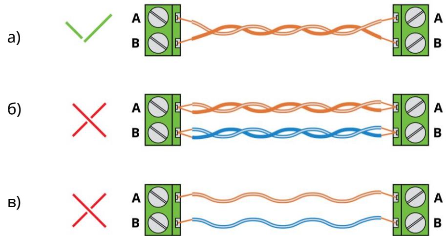
Рисунок 2.2 – Приклад підключення шини інтерфейсу RS-485
