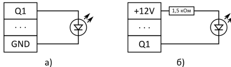
Рисунок 2.8 – Схеми підключення індикаторів підтвердження
