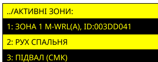
Рисунок 4.7 – Вікно зон модуля M-WRL(A) до яких приписані безпроводні сповіщувачі
