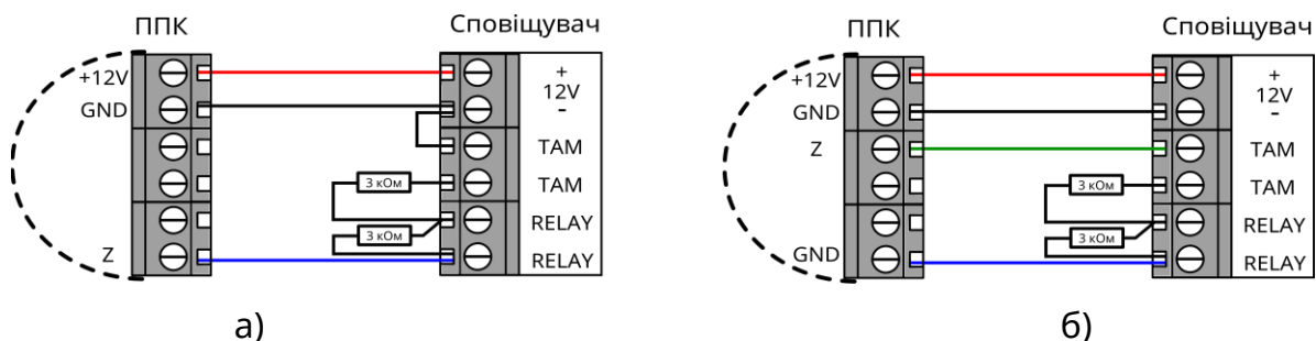
Рисунок 2.6 – Приклади підключення сповіщувачів по типу 2EOL
