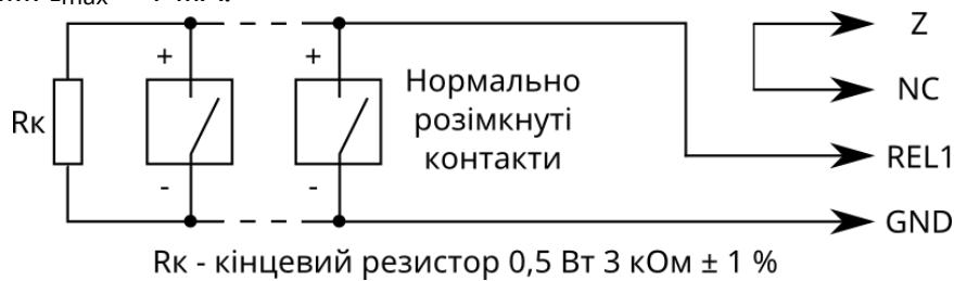
Рисунок 2.9 – Схема підключення двопровідних сповіщувачів з нормально розімкнутими контактами
