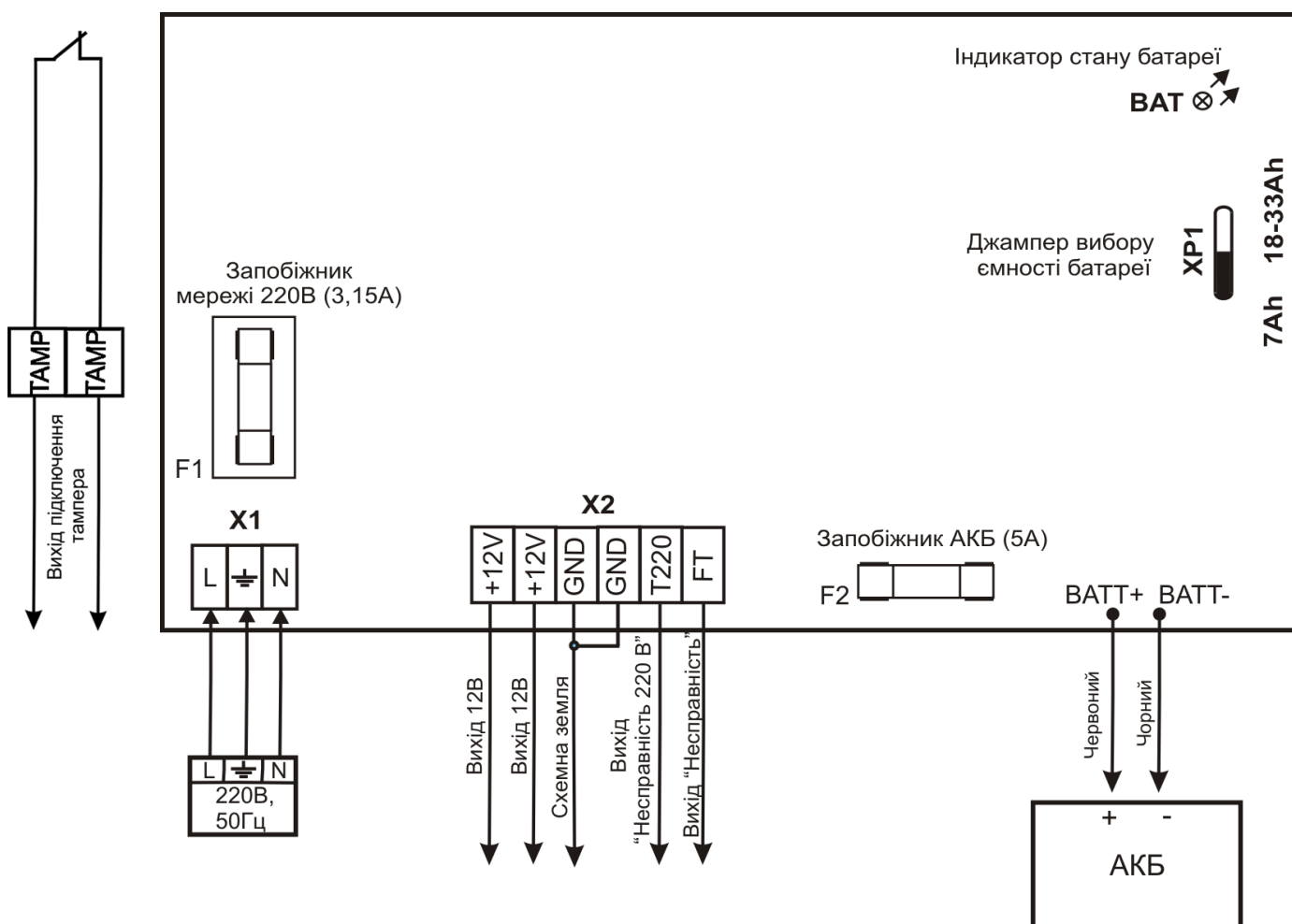
Рисунок А.2 – Підключення входів та виходів
