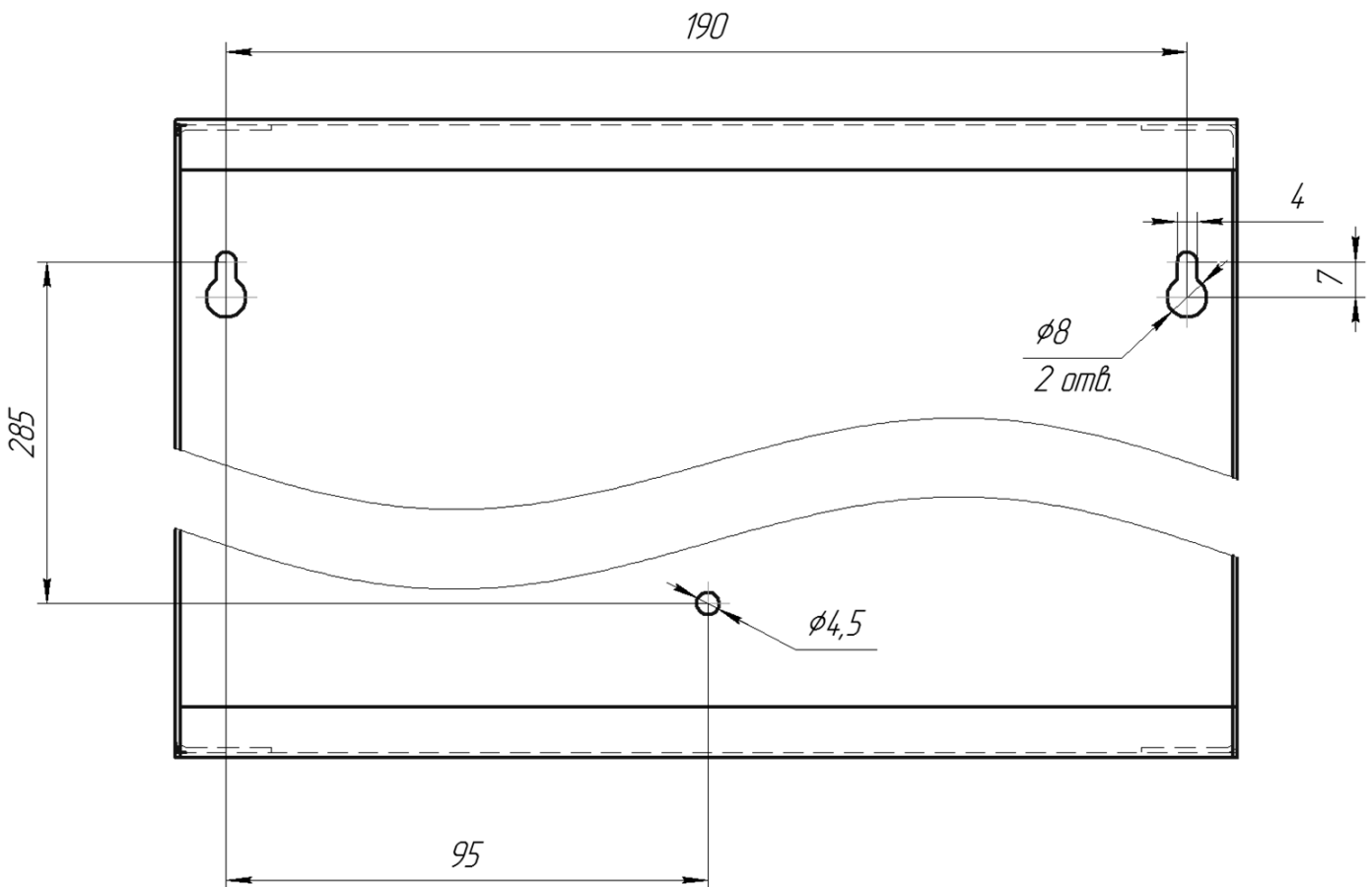
Рисунок Б.2 – Розмітка отворів для кріплення БЖ1220
