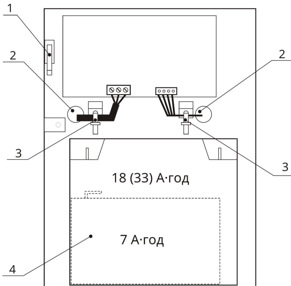
Рисунок В.1 – Компоновка БЖ:
