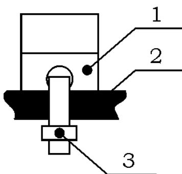
Рисунок В.2 – Спосіб кріплення проводів (рисунок В.1 поз. 3):
