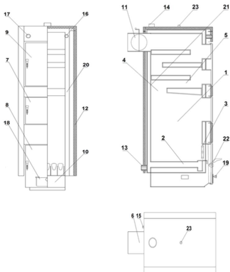
Рис. Котел SE
