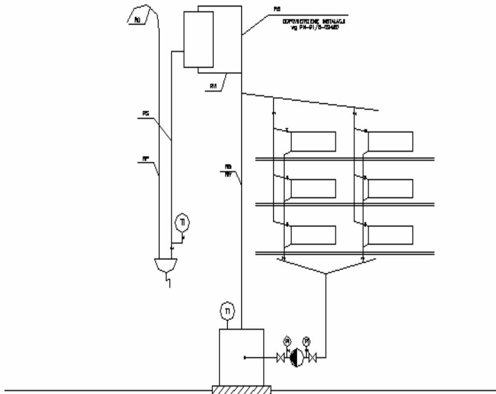
Рис. Схема защиты системы водяного отопления, оснащенного одним котлом, насос установлен на возврате (согласно PN-91/B-02413)
